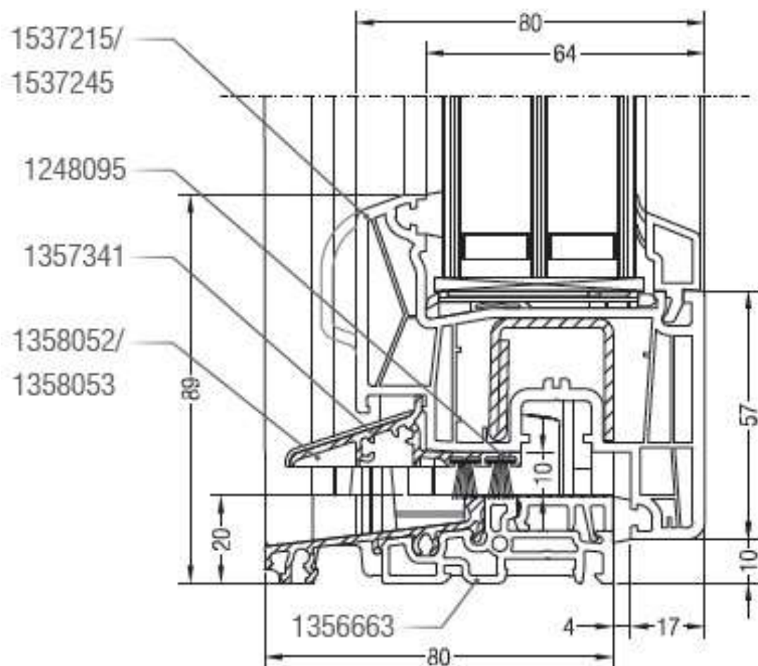
Sezione nodo anta arrotondata/dritta da 57 mm e soglia in Al
